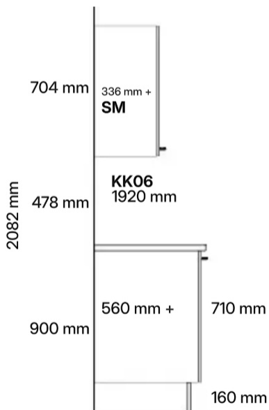
Kylkiprofiili 2082 mm
