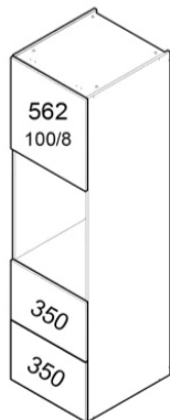
UUNI 2 LAATIKOLLA
