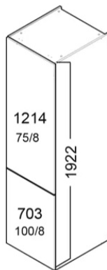
INTEGROITU JK/PK
